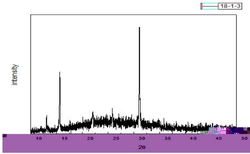
XRD
